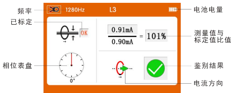
图 6-16 电缆识别界面
