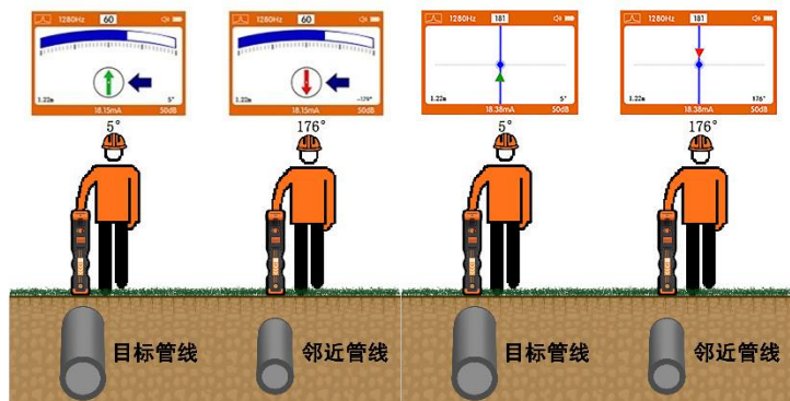
图 6-6 电流方向判定
