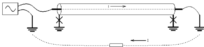
图 5-5 芯线-大地接法接线图
