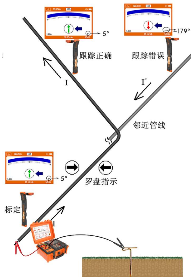
图 6-7 信号方向跟踪探测过程
