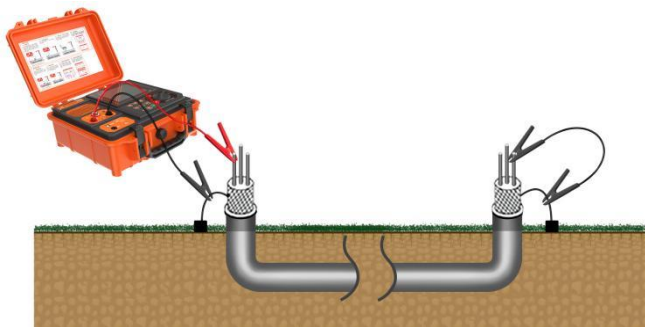
图 5-9 相线-护层接法接线图
