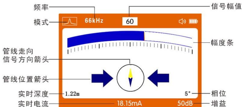
图 6-5 经典定位界面 (2)
