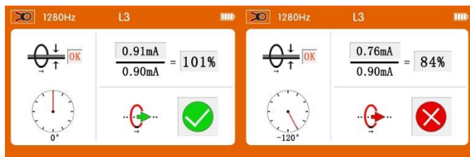
图 6-20 易对柔性线圈产生干扰区域
