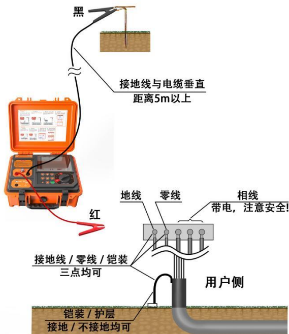
图 5- 21 运行电缆零线 / 地线 / 护层注入法
