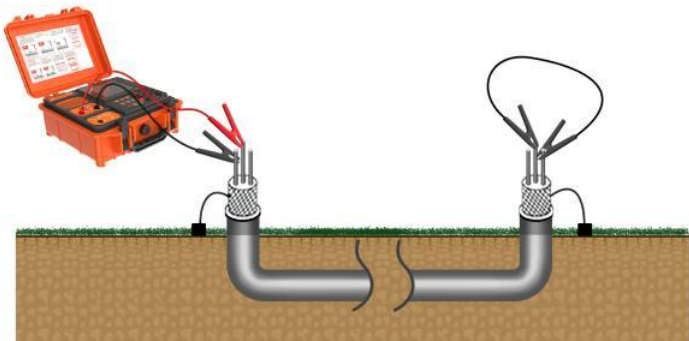
图 5- 12 相间接法接线图
