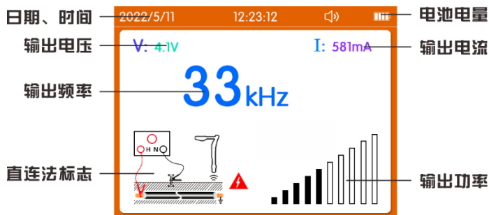
图 5-3 管线探测模式直连法输出界面图
