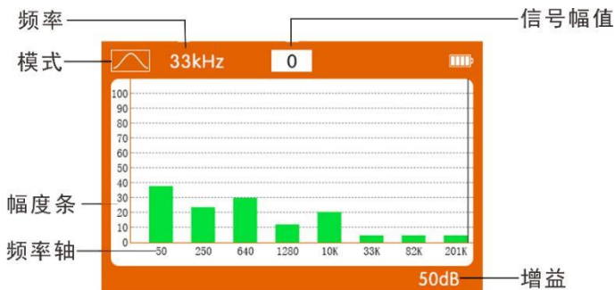
图 9-8 扫频测试界面
