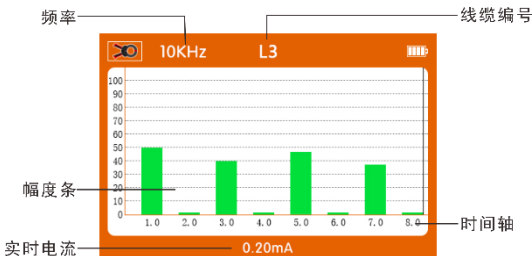
图 6- 2210kHz 以上的电缆识别界面
