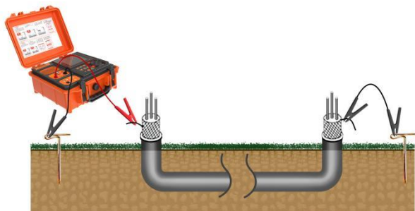
图 5-7 护层-大地接法接线图
