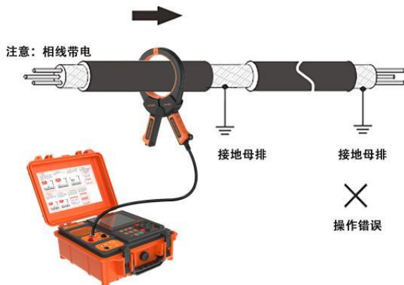
图 5-17 错误操作示范
