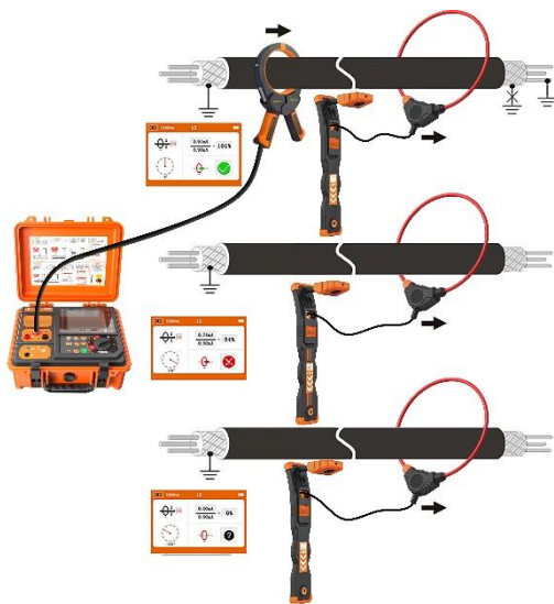
图 6-19 带电识别(耦合法)接线检测
