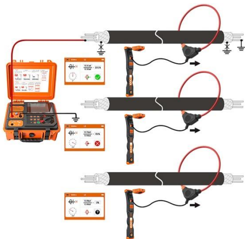
图 6-18 停电识别(直连法)接线检测
