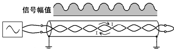
图 5-13 相间接法信号流向示意图
