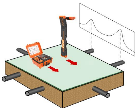
图 6-10 感应法区域探查
