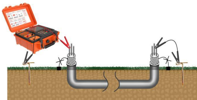
图 5-5 芯线-大地接法接线图
