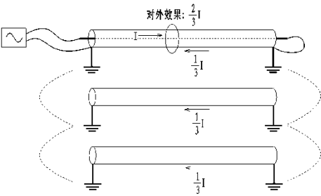
图 5- 11 并行电缆的分流效果
