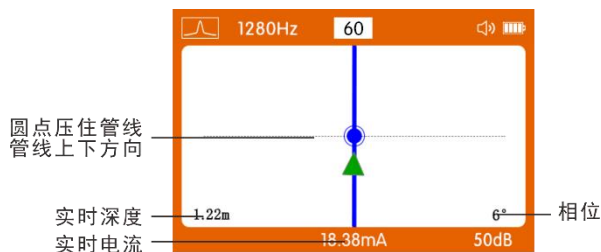
图 6-13 实时深度和电流测量
