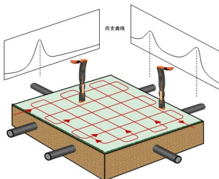
图 6-9 无源法区域探查
