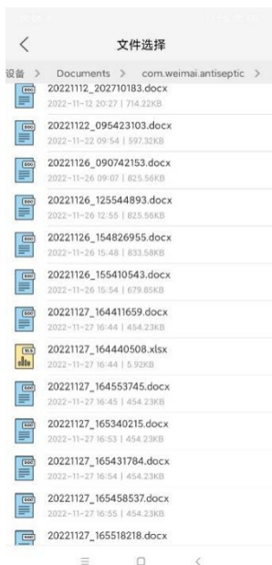
图 7-12 数据导入
